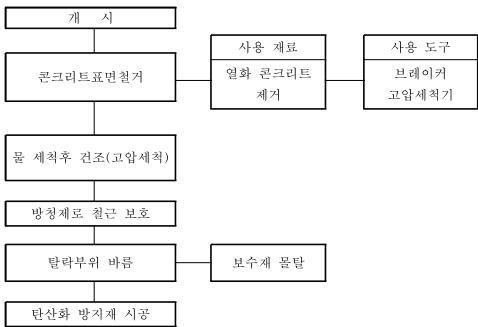
[단면복구공법 시공순서도]
