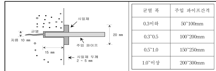
[균열 보수(주입공법) 개념도]
